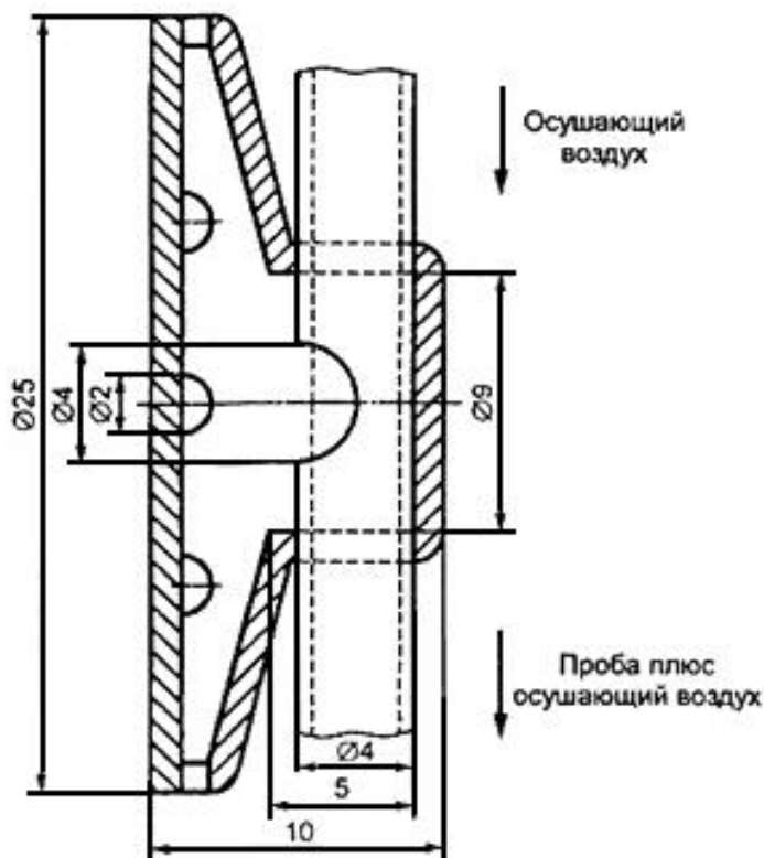
Рисунок 5 - Пробоотборник
